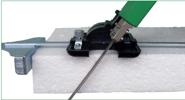
Führungsschlitten
