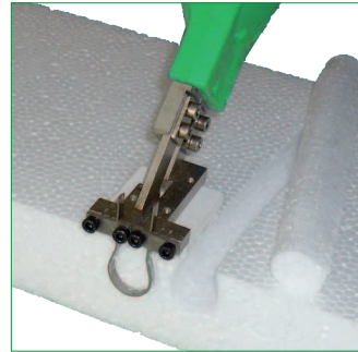
Nutenschneideschlitten klein
