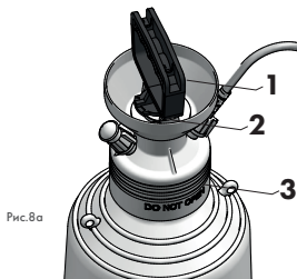
Рис.8а Поршневой шток не заблокирован
