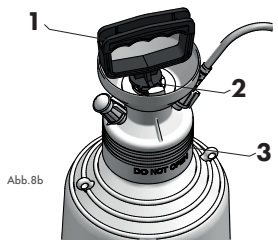
Kolbenstange verriegelt
