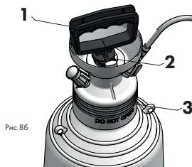
Поршневой шток заблокирован
